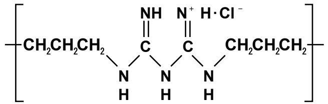
※ポリアミノプロピルビグアニドの構造式
